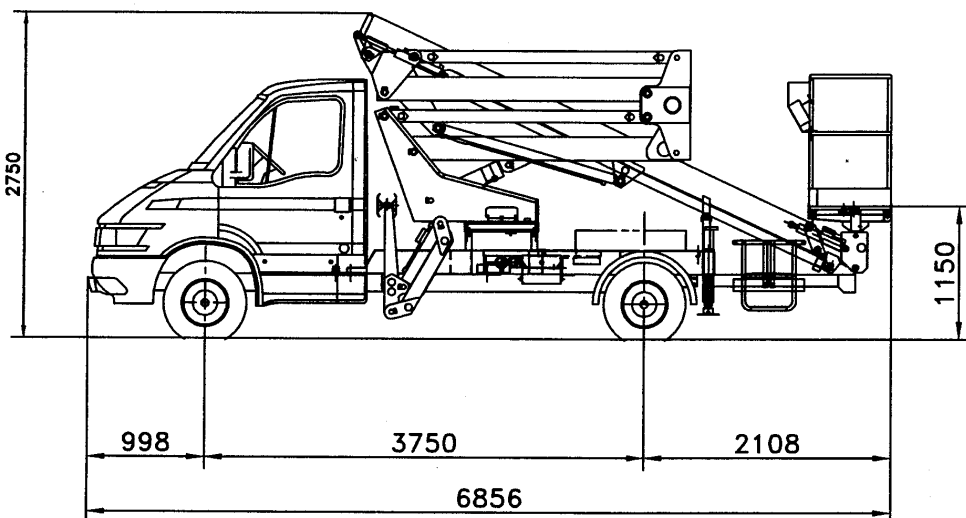
AUTOTELAIO IVECO 35 S
